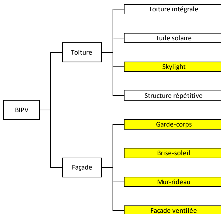
Figure 1: catégories BIPV
