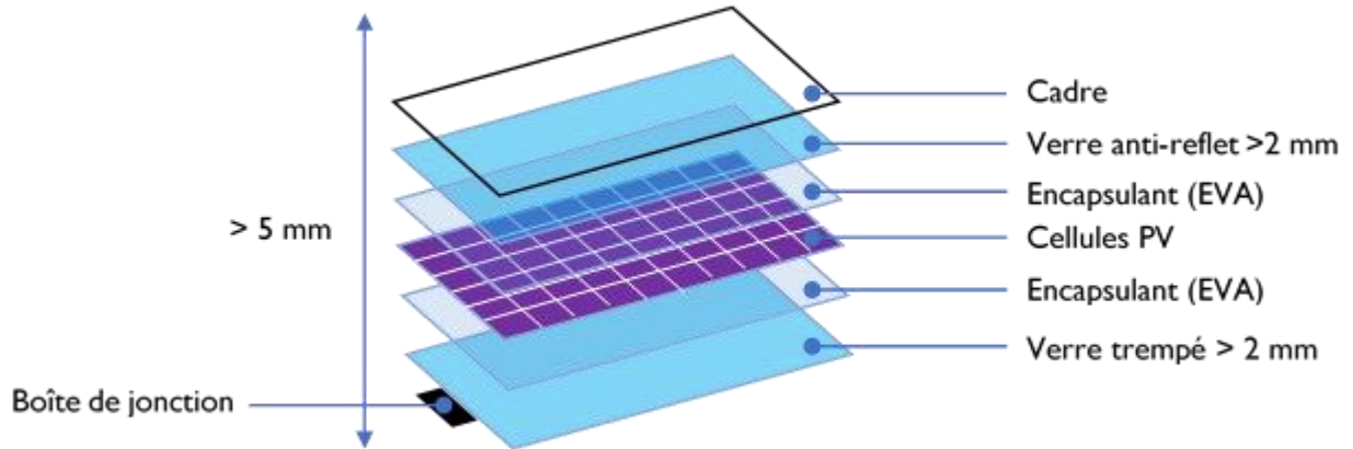
Figure 3: schéma d'un module photovoltaïque modifié
