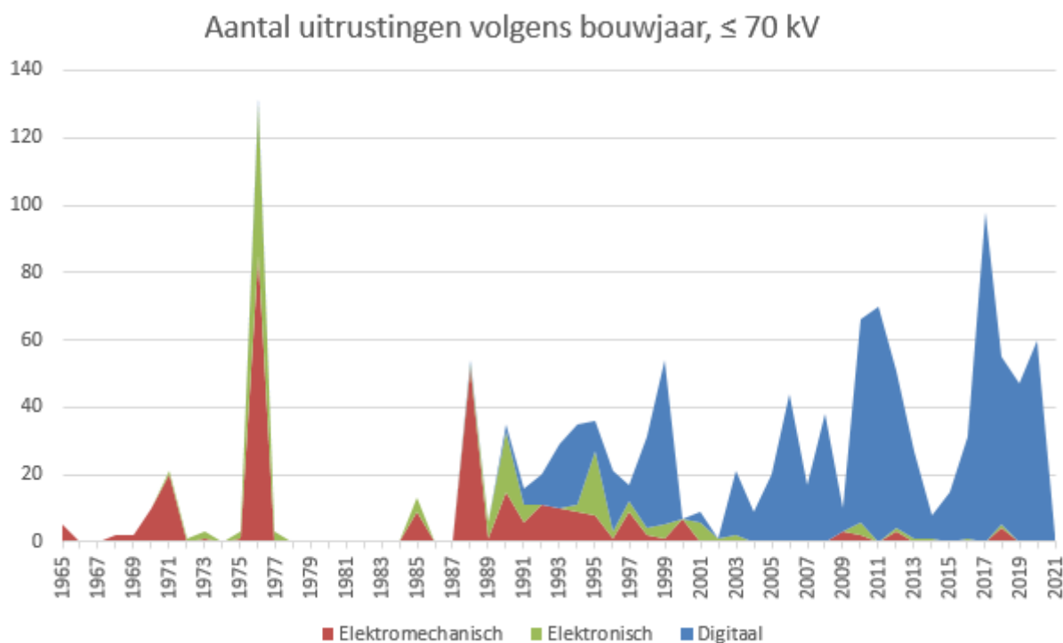
Figuur 2.5: Uitsplitsing van de beveiligingsuitrusting naar bouwjaar
